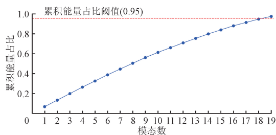
图 4 DMD 分解模态累积能量
