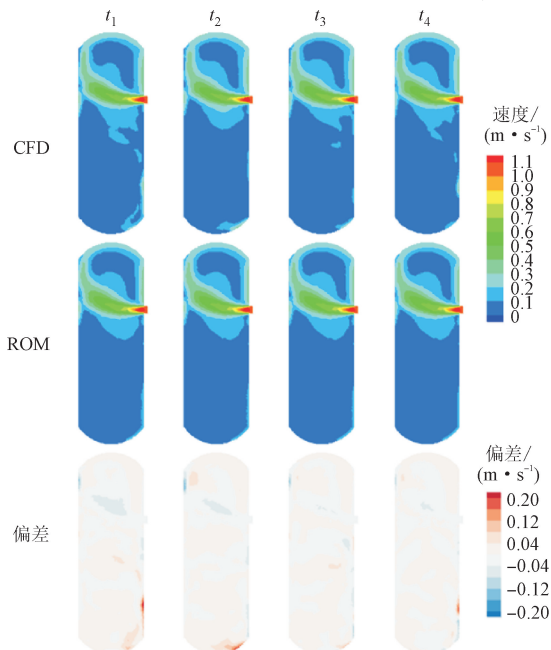
图 9 水蒸气的体积分数为 1% 工况下速度场 CFD 结果与 ROM 模型预测结果对比
