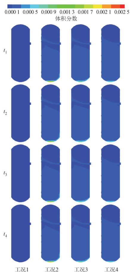
图6 不同工况下 ROM 模型预测结果
