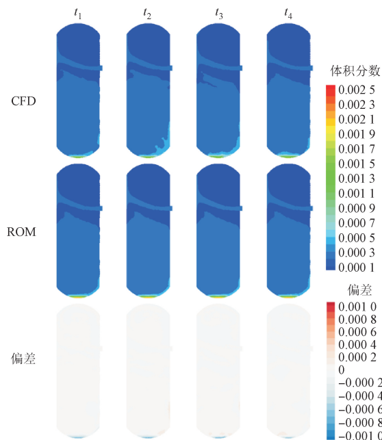
图7 水蒸气的体积分数为 1% 工况下水的体积分数的场分布 CFD 结果与 ROM 模型预测结果对比
