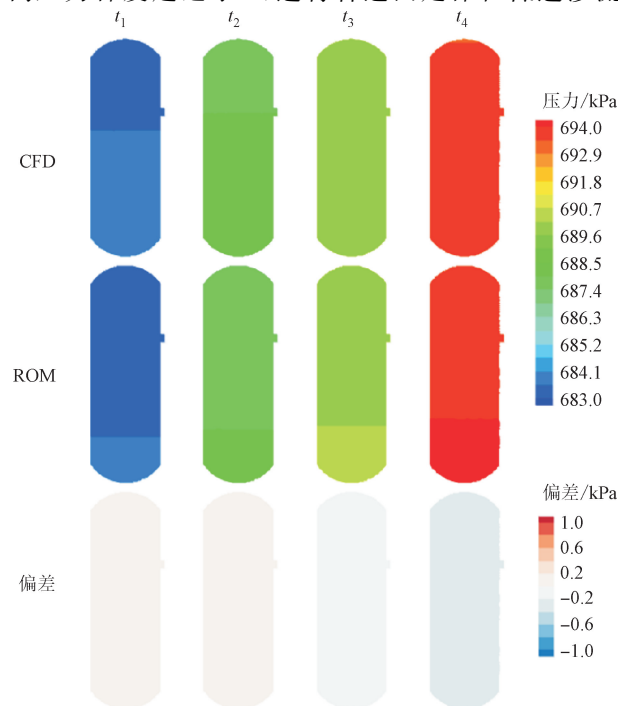
图10 水蒸气的体积分数为1%工况下压力场CFD结果与ROM模型预测结果对比
