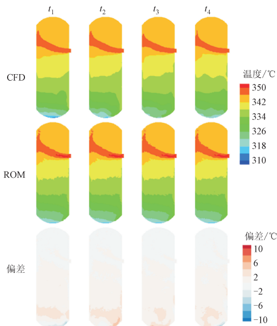
图 8 水蒸气的体积分数为 1% 工况下温度场 CFD 结果与 ROM 模型预测结果的对比
