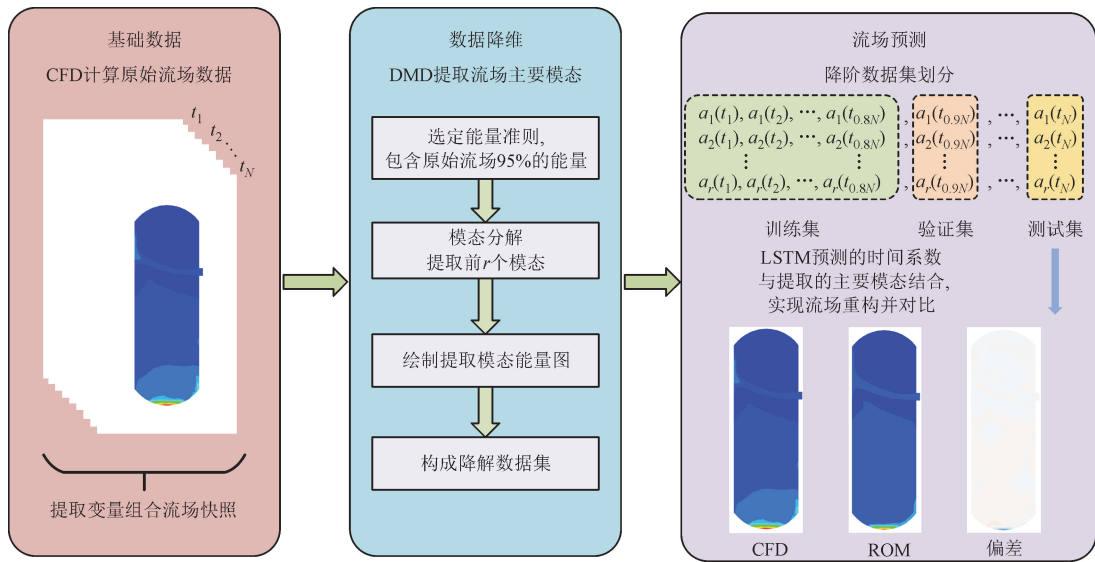
图 3 DMD-LSTM 混合降阶模型程序流程框架
