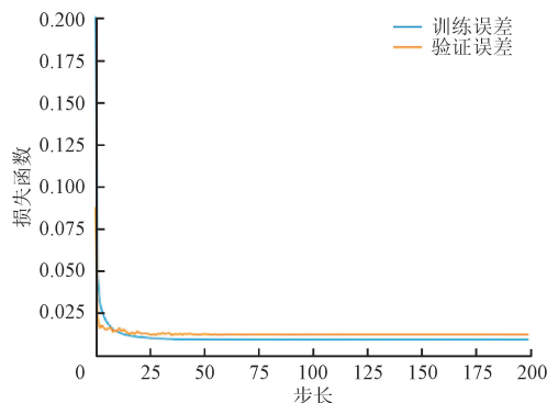
图 5 LSTM 模型训练损失函数
